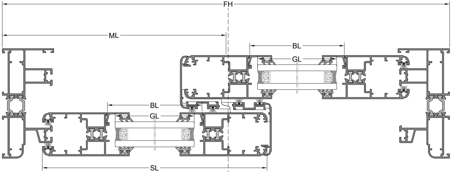
A-A KESİTİ
