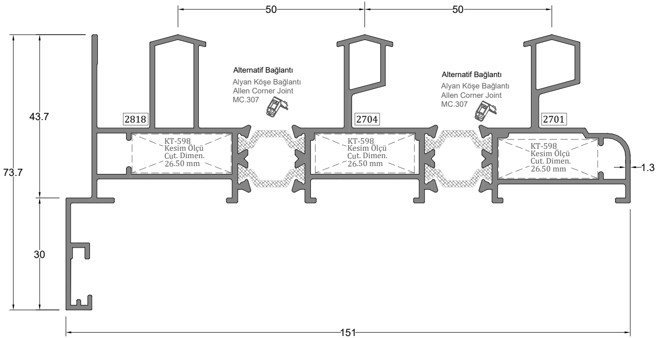
Üç Raylı Kasa Profili TRIPLE RAIL FRAME PROFILE
