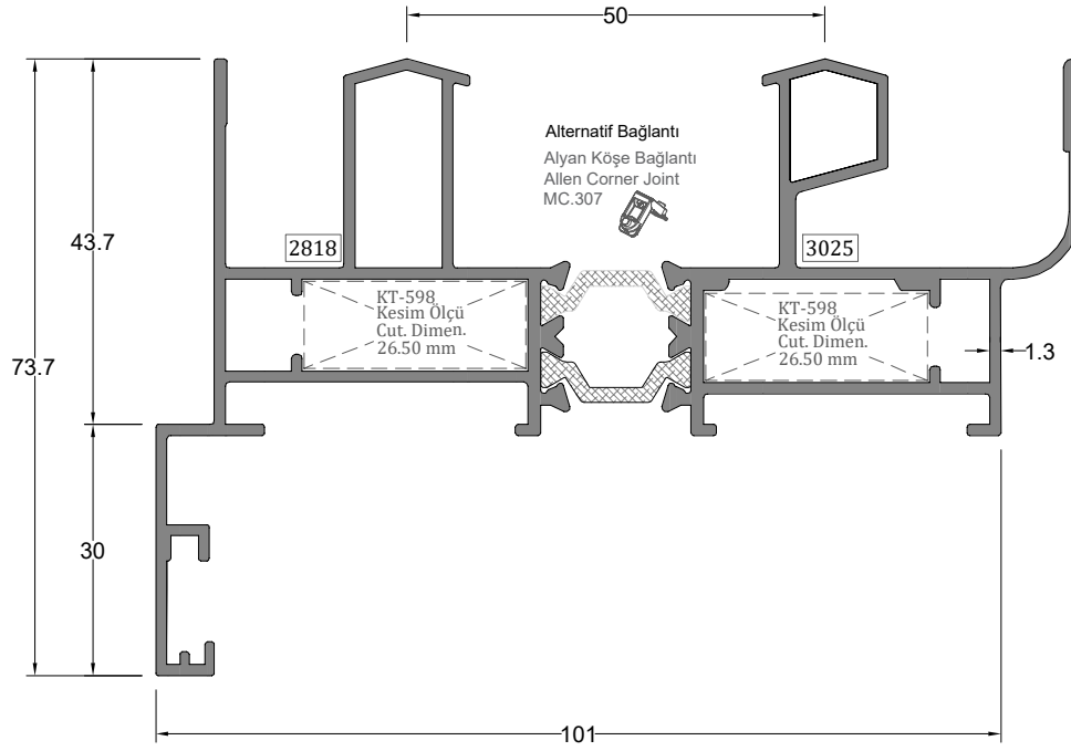
İki Raylı Sineklikli Kasa Profili DOUBLE RAIL SCREENING FRAME PROFILE
