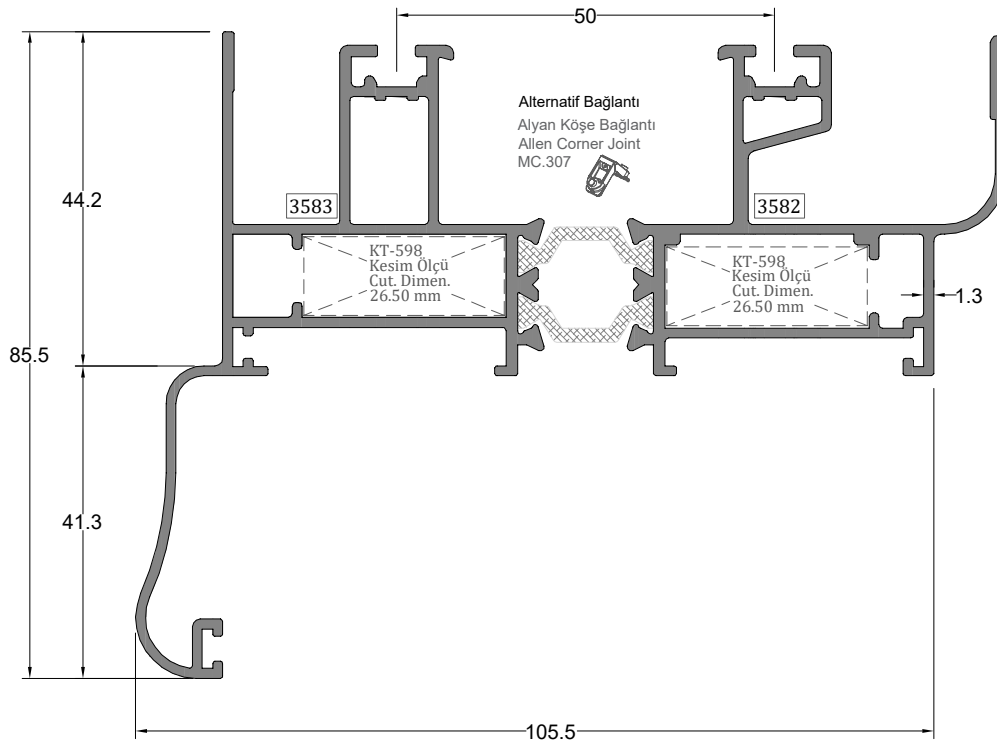
İki Raylı Sineklikli Kasa Profili DOUBLE RAIL SCREENING FRAME PROFILE
