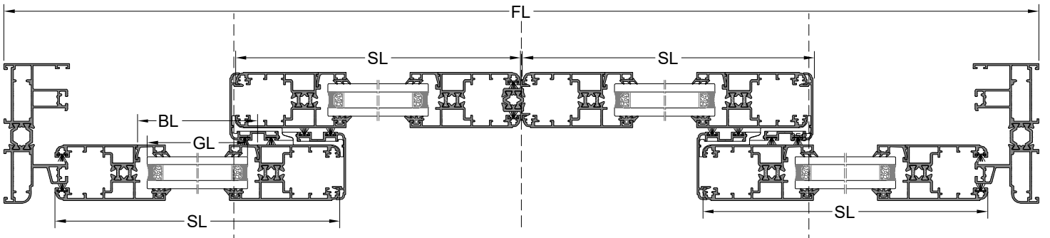
A-A KESİTİ
