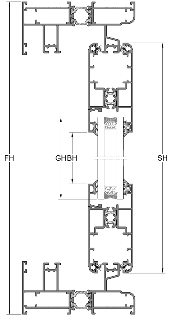
B-B KESİTİ
