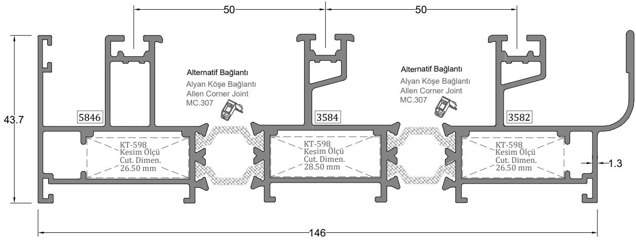
Üç Raylı Sineklikli Kasa Profili TRIPLE RAIL SCREENING FRAME PROFILE
